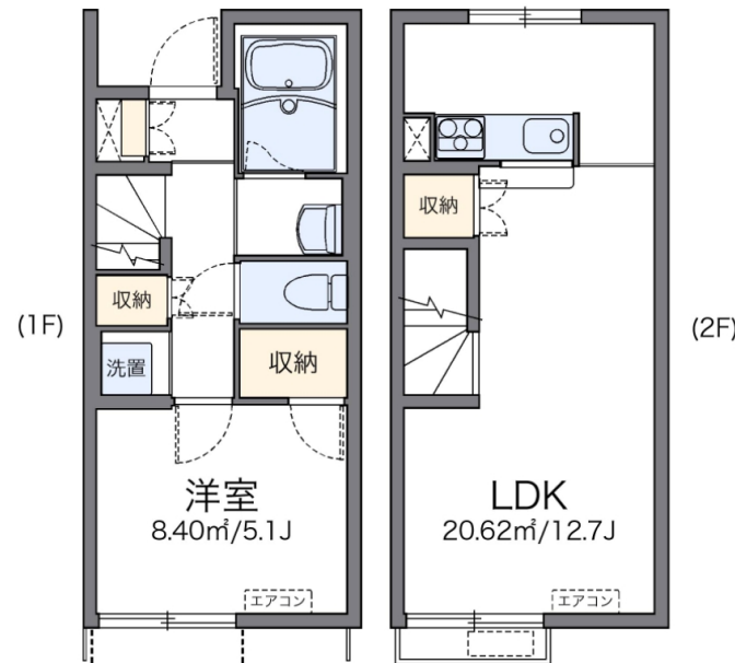
【間取り図】
