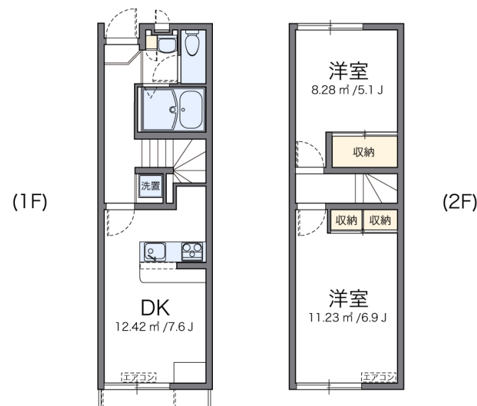
【間取り図】
