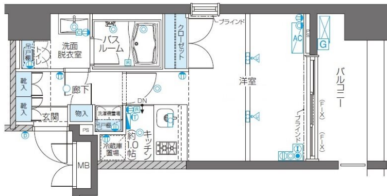
ZOOM目黒/平面詳細図/Eタイプ
