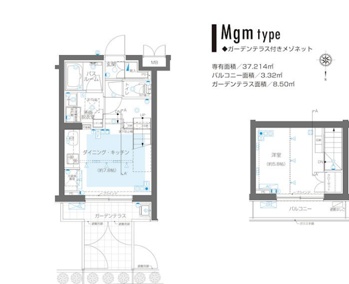
【間取り図】
