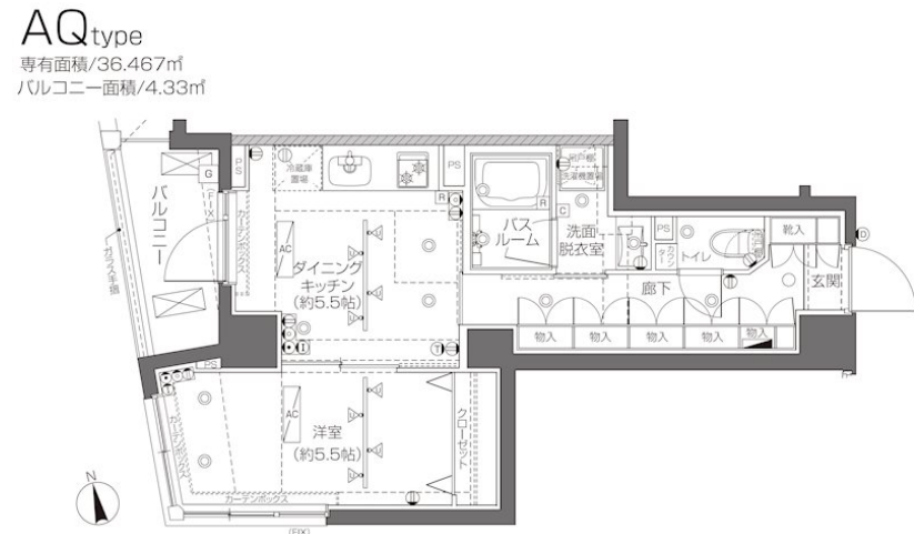
【間取り図】
